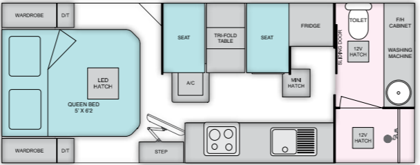
VAN 4 - 19'8"
