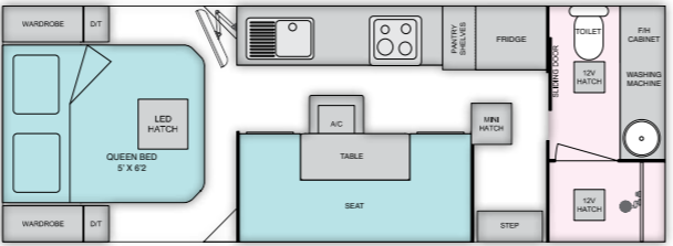
VAN 7 CLUB- 21'6"
