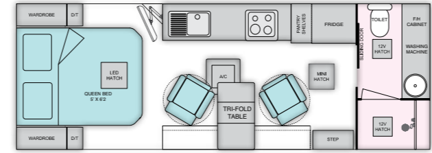
VAN 7 RECLINER - 21'6"
