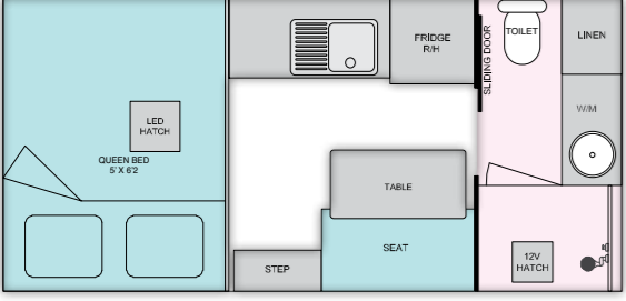
VAN 1C - 15'
