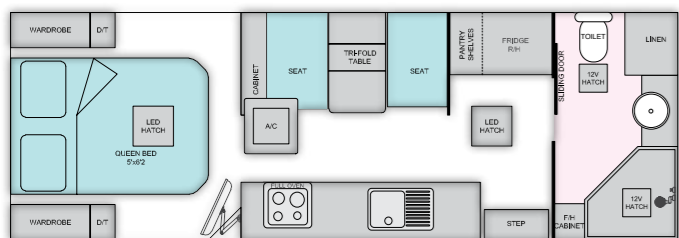
VAN 9 - 21'10"
