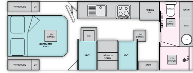
VAN 5 - 20'
