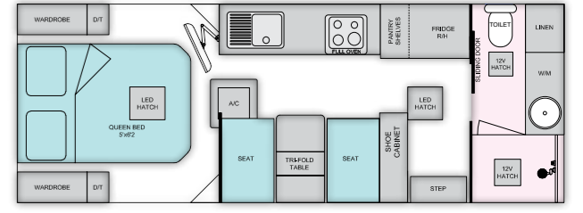
VAN 5-2 - 20'6"
