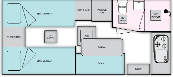
VAN 1F - 16'
