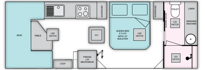
VAN 8 CLUB - 21'10"
